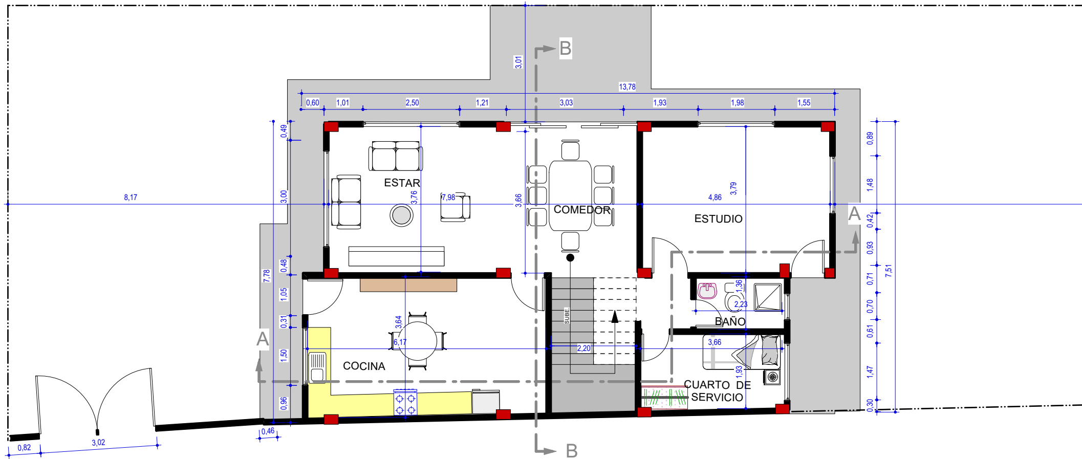
PLANTA BAJA Y EMPLAZAMIENTO
